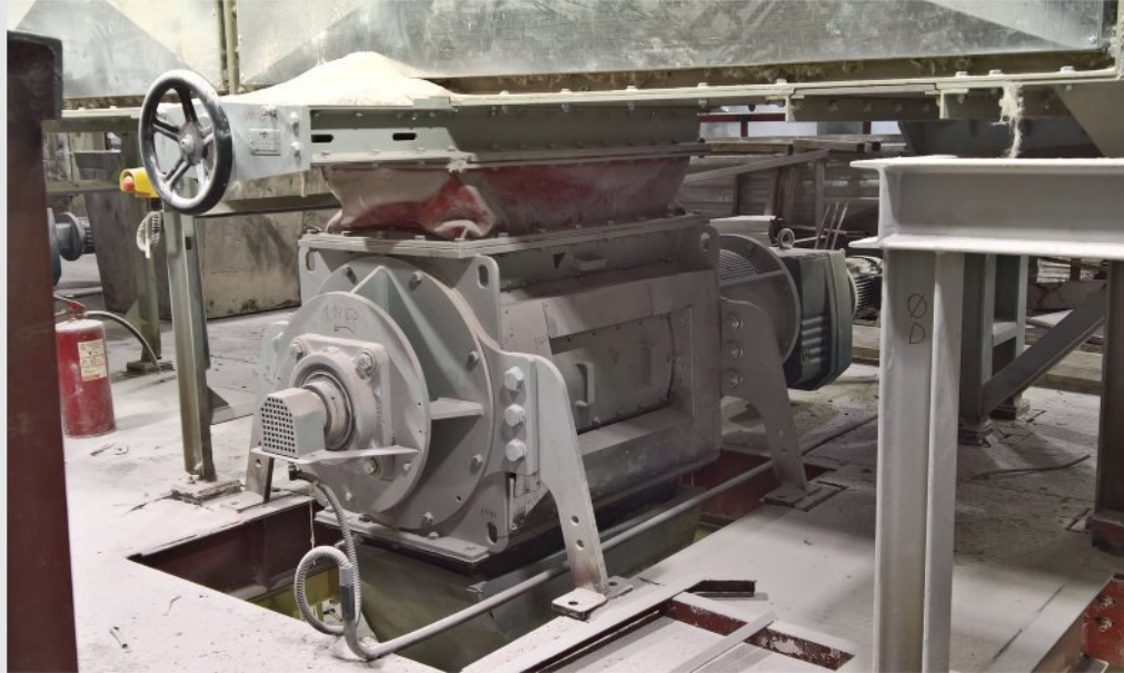
Zellenradschleuse in der Kaliindustrie
