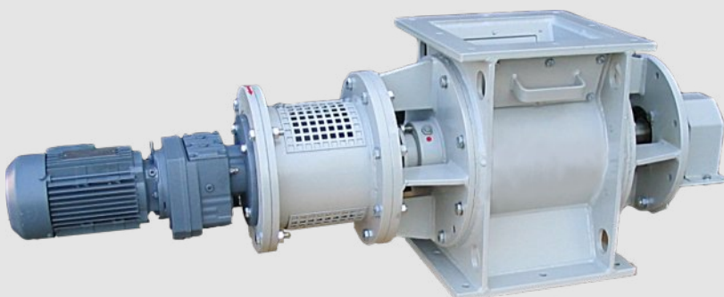
Zellenradschleuse mit Getriebemotor
