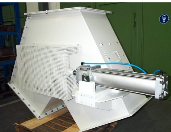
Wegeverteiler pneumatisch
